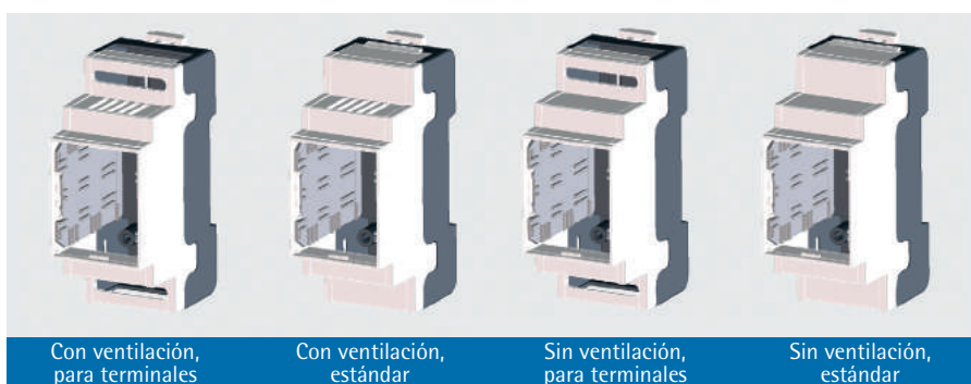
Variantes abiertas para panel frontal (p.ej. Caja DB 2 Módulos)
