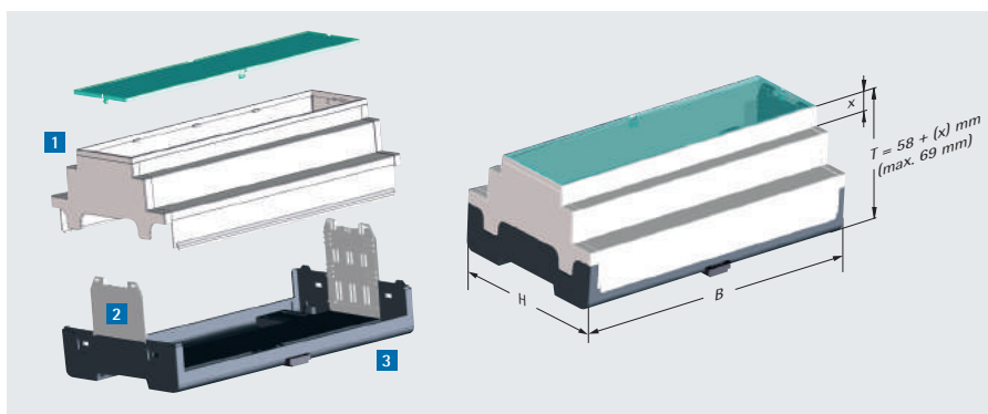
Variantes cerradas (p.ej. Caja DB 2 Módulos)
