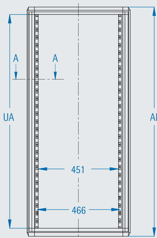
Dimensiones del armario y medidas de montaje
