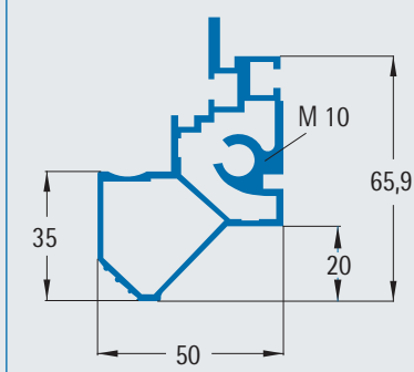
Sección del perfil A-A
