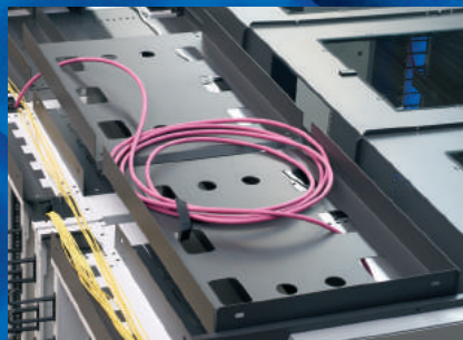
Bandeja de cableado superior
