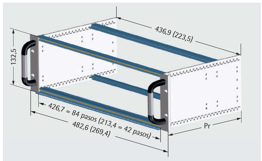
Posibilidad de montaje con extractor de tarjeta y placa BUS / con asas
